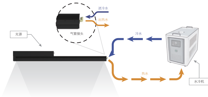
附录1: 超高亮线光源冷却系统结构示意图
