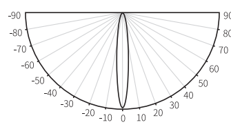
配光特性:短边方向
